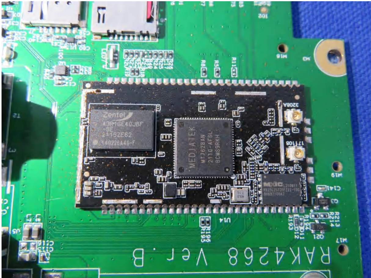
BLE module RAK13400
