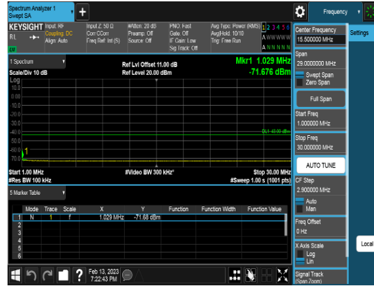
Port1_10M_3555MHz_TM3.2_CHL_CSE2
