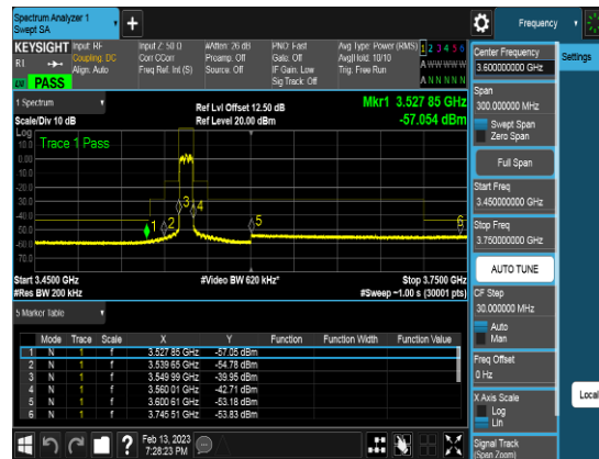
Port1_10M_3555MHz_TM3.2_CHL_CSEpart96
