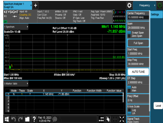
Port2_20M_3690MHz_TM3.1_CHH_CSE2
