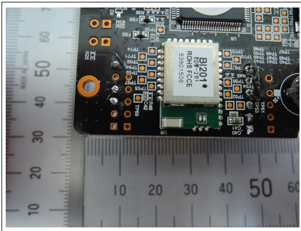
<BLE Antenna>
