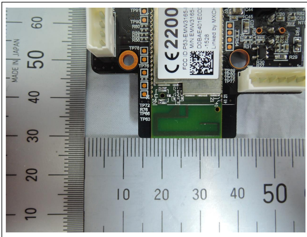
<WLAN Antenna>
