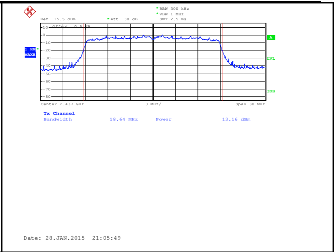
Output power - Mid CH 2437 - 802.11 n(20M)
