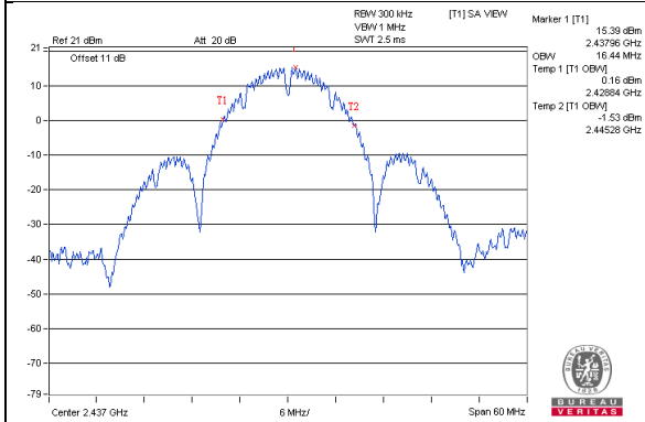
VHT20 / Chain 2 : CH6
