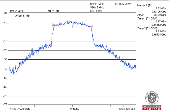
VHT40 / Chain 2 : CH6
