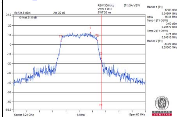
802.11a_Chain 1 / CH48
