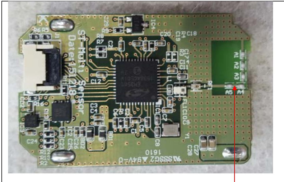
Antenna
