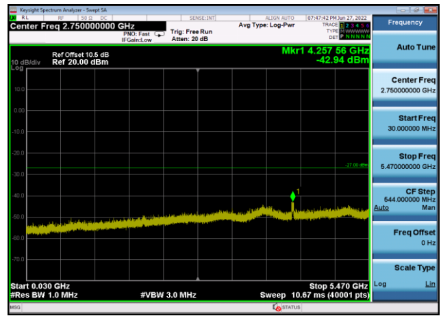
U-NII-2c ,Plot 2,30MHz~5470MHz-802.11 ac(80MHz),5610MHz,Ant1
