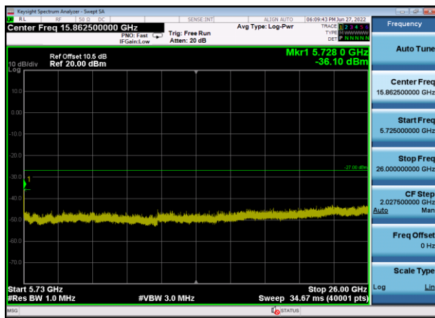
U-NII-2c ,Plot 3,5725MHz~26000MHz-802 .11ac(20MHz),5600MHz,Ant1
