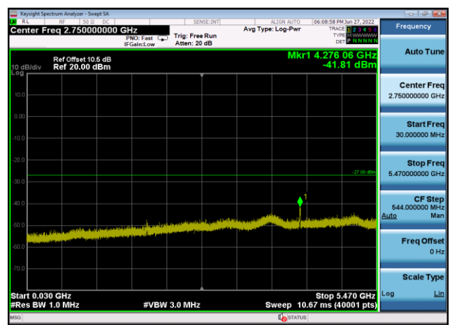
U-NII-2c ,Plot 2,30MHz~5470MHz-802.11 ac(20MHz),5600MHz,Ant1
