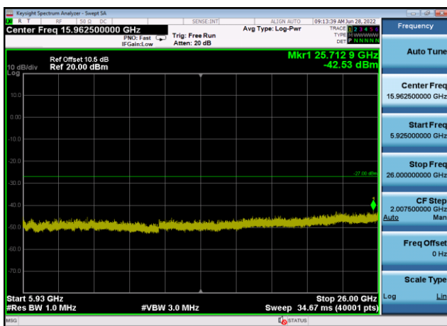
U-NII-3 ,Plot 3,5925MHz~26000MHz-802.11n(20MHz),5785MHz,Ant1
