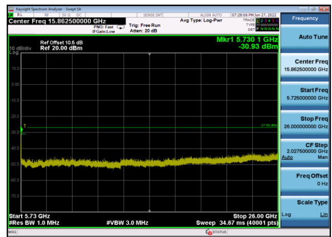
U-NII-2c ,Plot 3,5725MHz~26000MHz-802 .11ac(40MHz),5590MHz,Ant1
