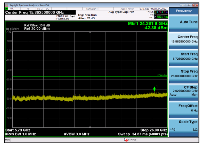
U-NII-2c ,Plot 3,5725MHz~26000MHz-802 .11ac(20MHz),5700MHz,Ant1
