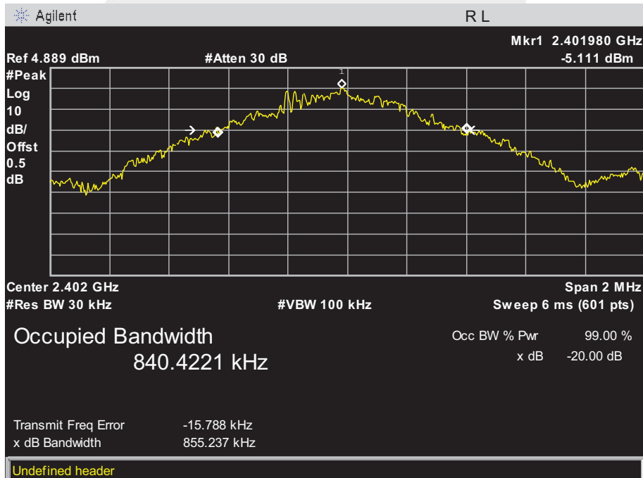
CH00 -1Mbps
