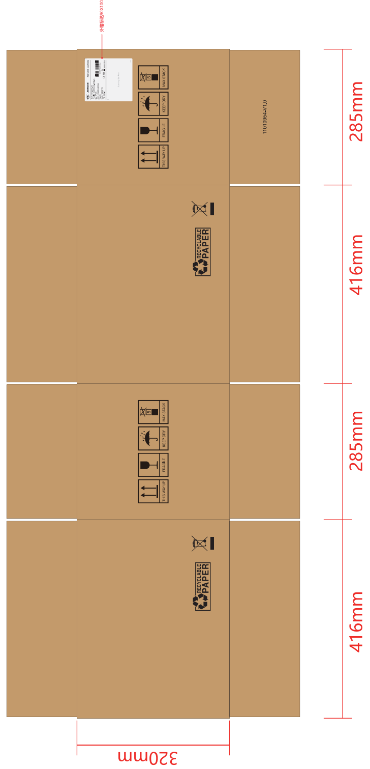
外箱标贴位置示意
