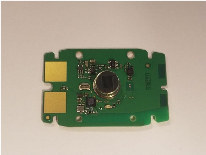
PCB bottom
