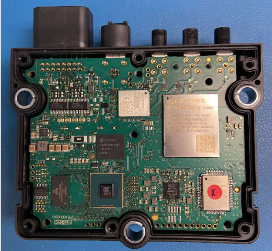
Appareo Parshall - USA Model—Internal Photos
