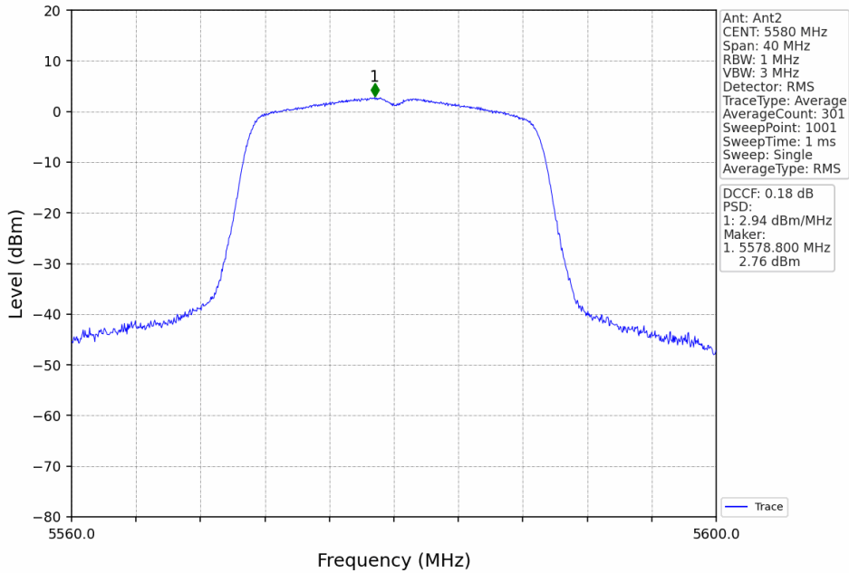
802.11n(HT20)_MCH_5580MHz_MIMO_NTNV
