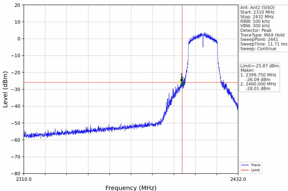
802.11g_LCH_2412MHz_Ant2 (SISO)_NTNV
