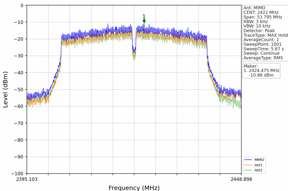
802.11n(HT40)_LCH_2422MHz_MIMO_NTNV
