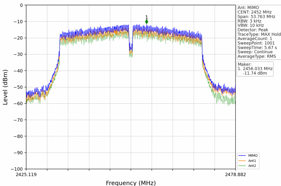
802.11n(HT40)_HCH_2452MHz_MIMO_NTNV
