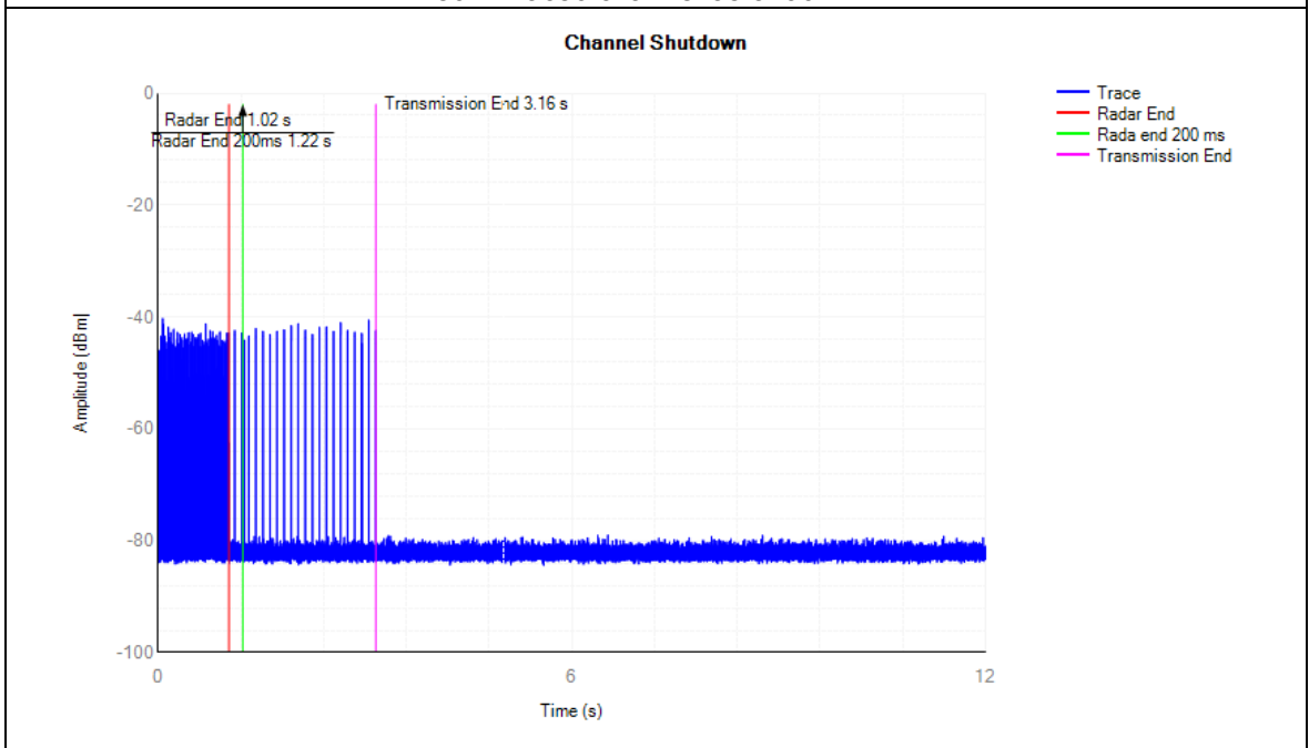
802.11ac80 channel 106 5530MHz
