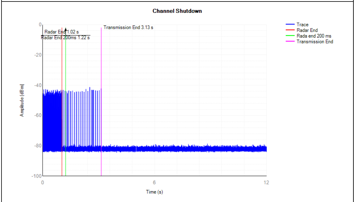
802.11n40 channel 102 5510MHz
