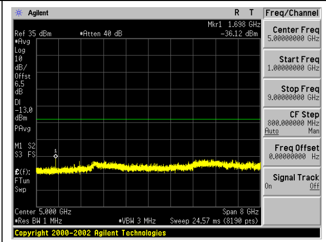
GSM 850-HCH
