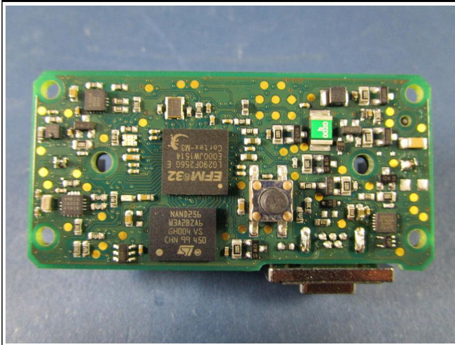
EUT-PCB Bottom
