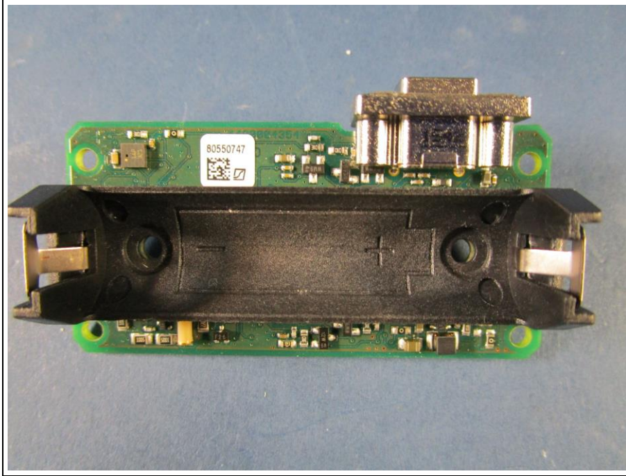
EUT-PCB Top
