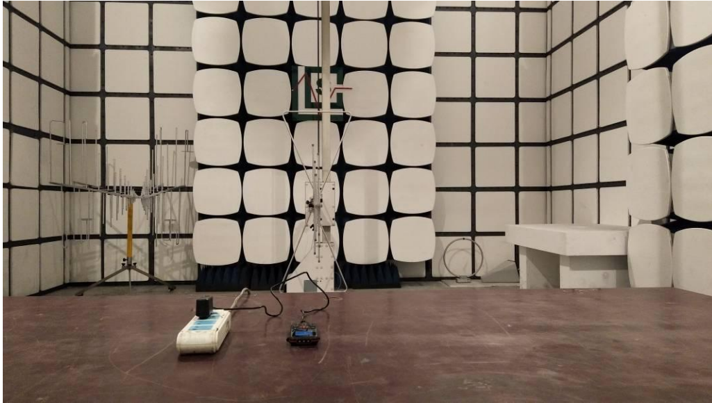
Fig. 1 (Below 1GHz)
