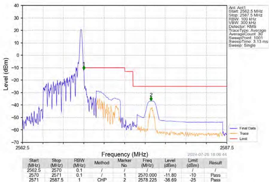
Band7 5MHz 16QAM HCH 2567.5MHz RB 1 24 NTV
