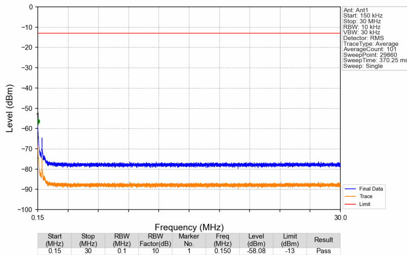
Band26b_869.1MHz_GMSK_SISO_Ant1_NTNV
