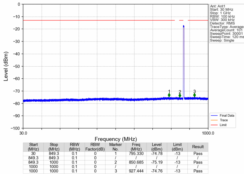
Band26b_871.5MHz_AWGN_SISO_Ant1_NTNV
