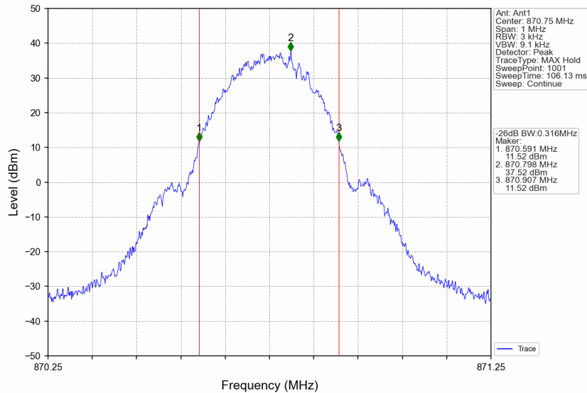
Band26b_870.75MHz_GMSK_SISO_Ant1_NTNV_AGC
