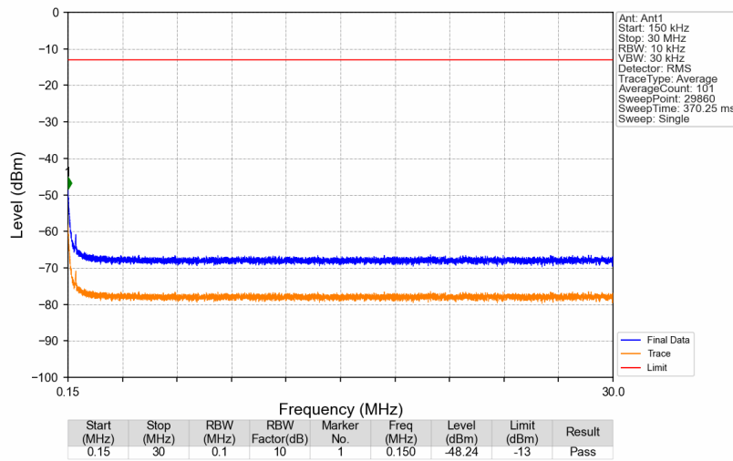
Band26b_881.5MHz_AWGN_SISO_Ant1_NTNV
