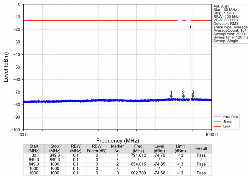
Band26b_891.5MHz_AWGN_SISO_Ant1_NTNV
