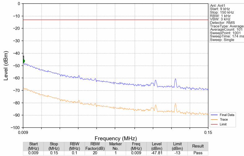
Band26b_893.9MHz_GMSK_SISO_Ant1_NTNV
