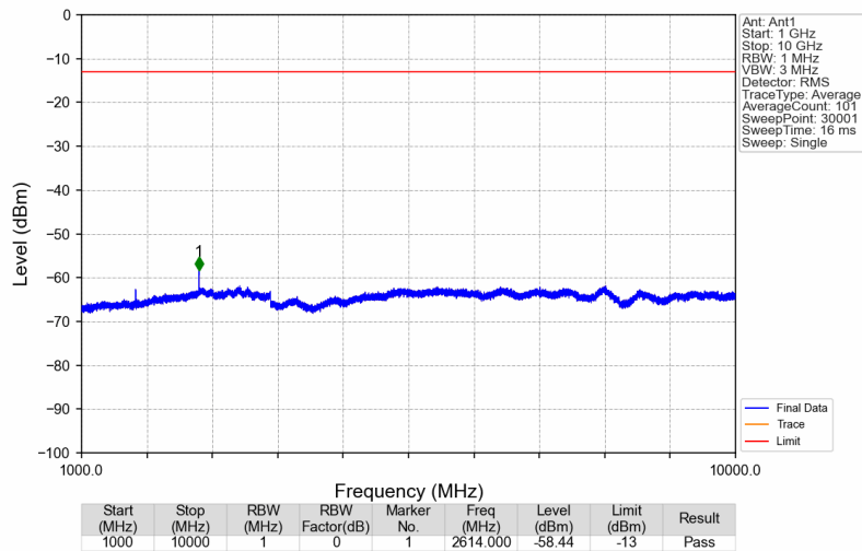
Band26b_871.5MHz_AWGN_SISO_Ant1_NTNV
