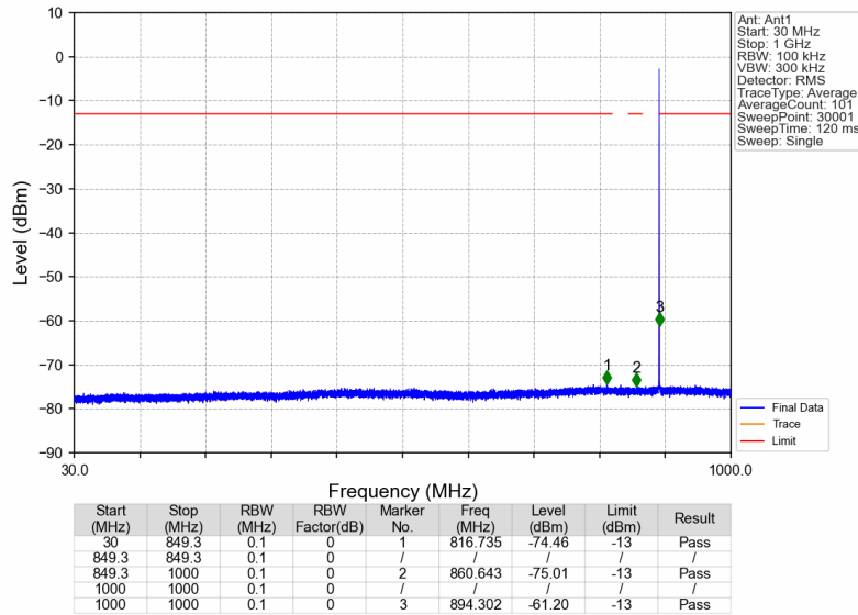
Band26b_893.9MHz_GMSK_SISO_Ant1_NTNV
