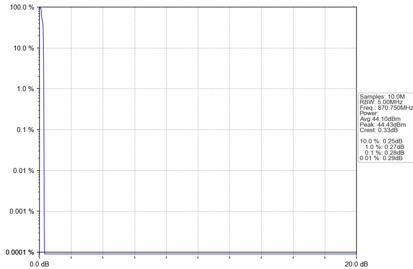
Band26b_870.75MHz_GMSK_SISO_Ant1_NTNV_AGC+3
