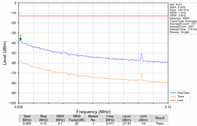
Band26b_881.5MHz_GMSK_SISO_Ant1_NTNV
