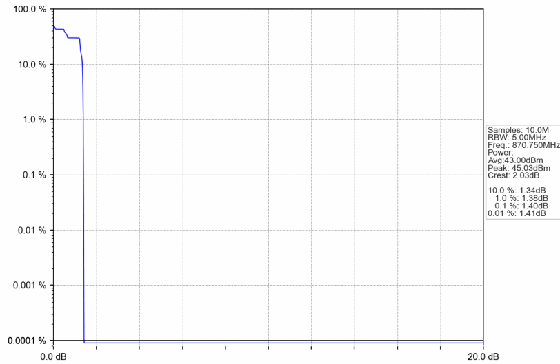
Band26b_870.75MHz_GMSK_SISO_Ant1_NTNV_AGC
