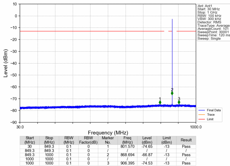
Band26b_869.1MHz_GMSK_SISO_Ant1_NTNV
