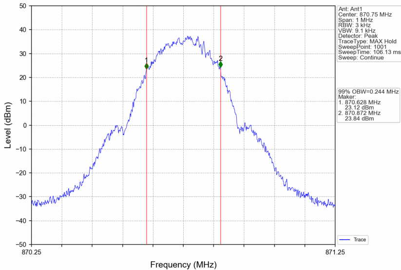
Band26b_870.75MHz_GMSK_SISO_Ant1_NTNV_AGC
