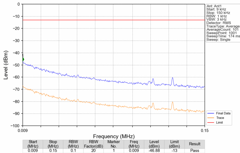
Band26b_891.5MHz_AWGN_SISO_Ant1_NTNV
