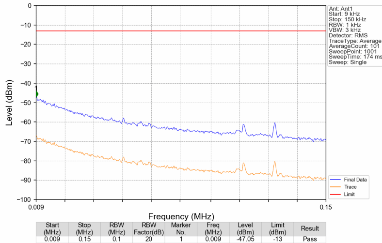
Band26b_869.1MHz_GMSK_SISO_Ant1_NTNV
