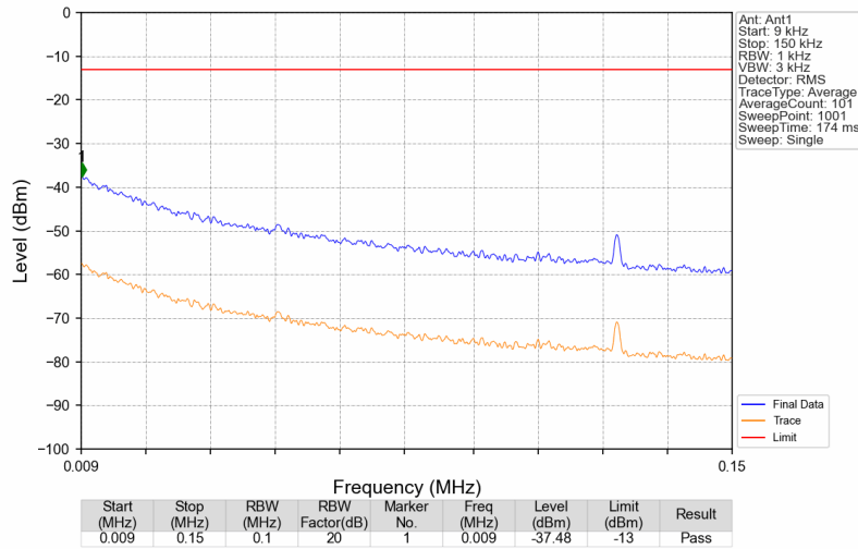
Band26b_881.5MHz_AWGN_SISO_Ant1_NTNV
