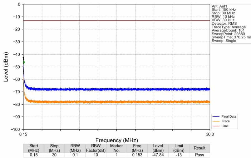
Band26b_881.5MHz_GMSK_SISO_Ant1_NTNV
