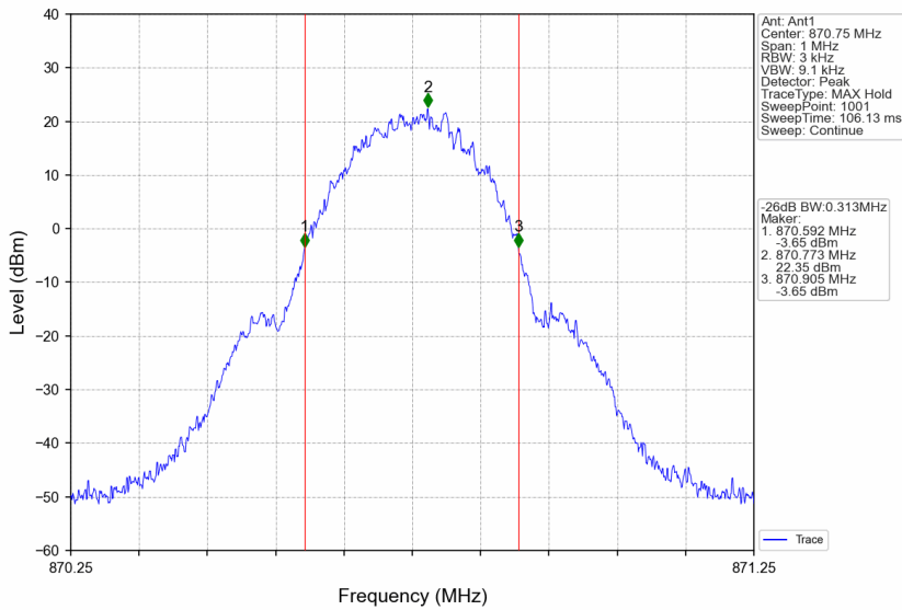
Band26b_870.75MHz_GMSK_SISO_Ant1_NTNV_AGC+3
