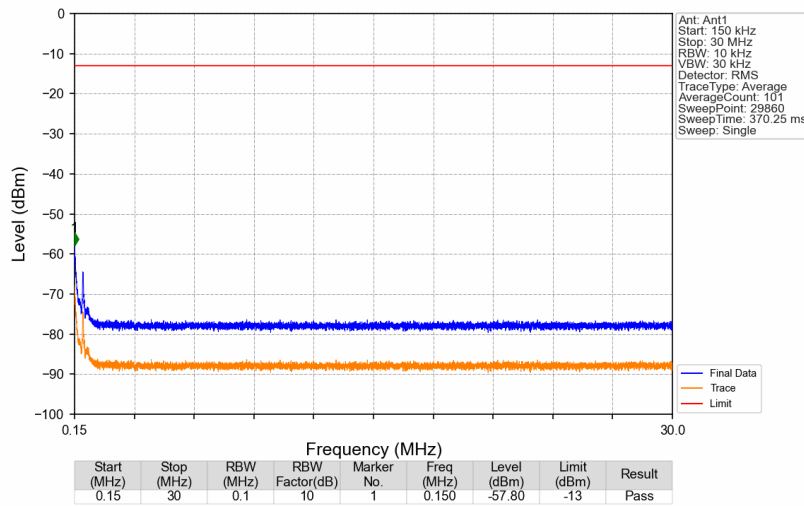
Band26b_893.9MHz_GMSK_SISO_Ant1_NTNV
