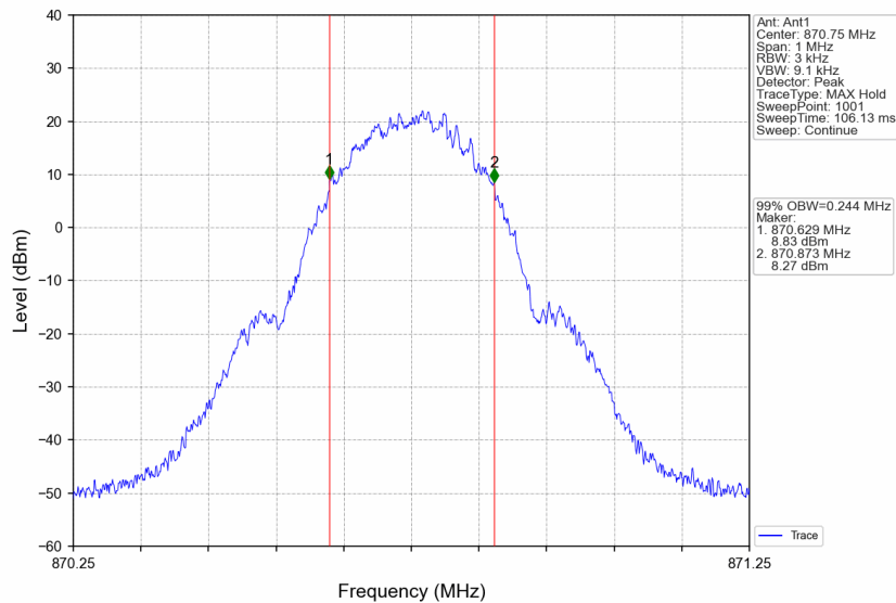
Band26b_870.75MHz_GMSK_SISO_Ant1_NTNV_AGC+3
