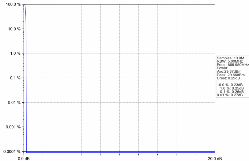
Band26a_866.95MHz_GMSK_SISO_Ant1_NTNV_AGC+3
