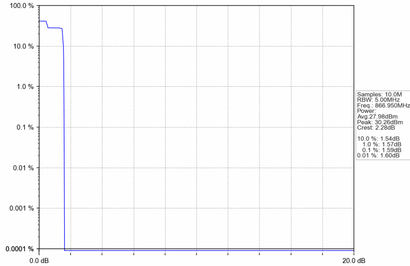
Band26a_866.95MHz_GMSK_SISO_Ant1_NTNV_AGC
