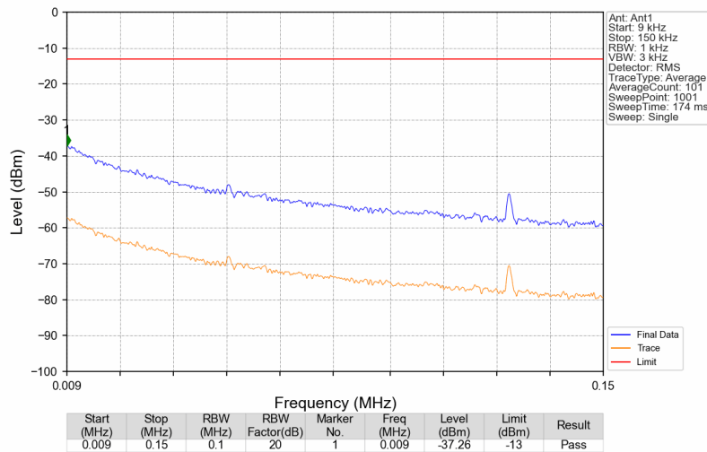
Band26a_868.9MHz_GMSK_SISO_Ant1_NTNV
