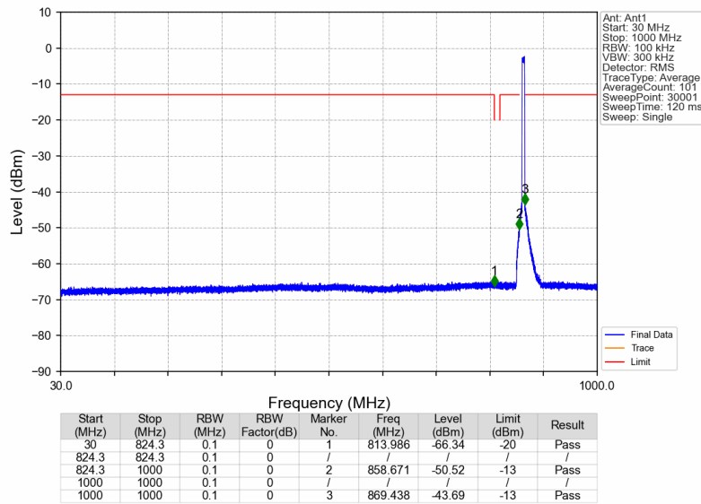
Band26a_866.5MHz_AWGN_SISO_Ant1_NTNV
