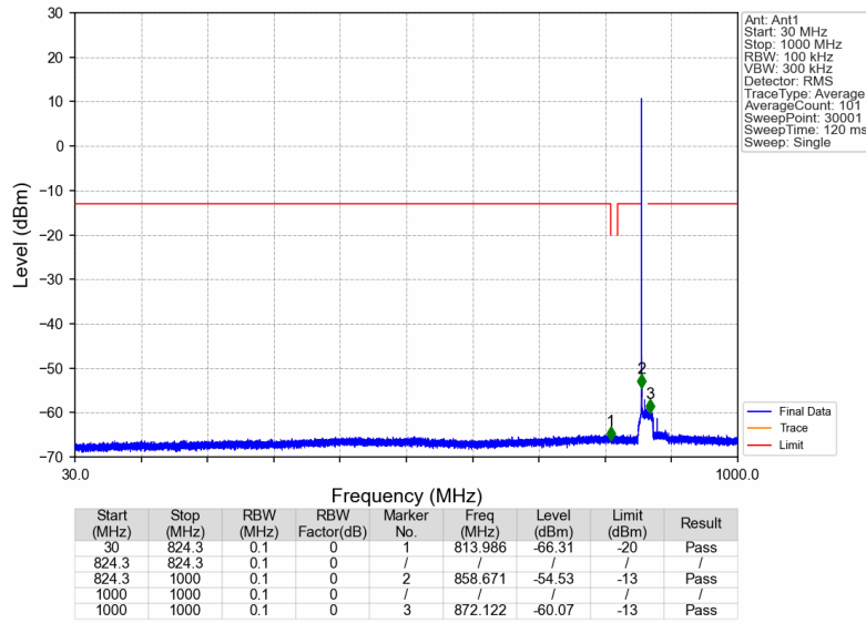
Band26a_859.1MHz_GMSK_SISO_Ant1_NTNV
