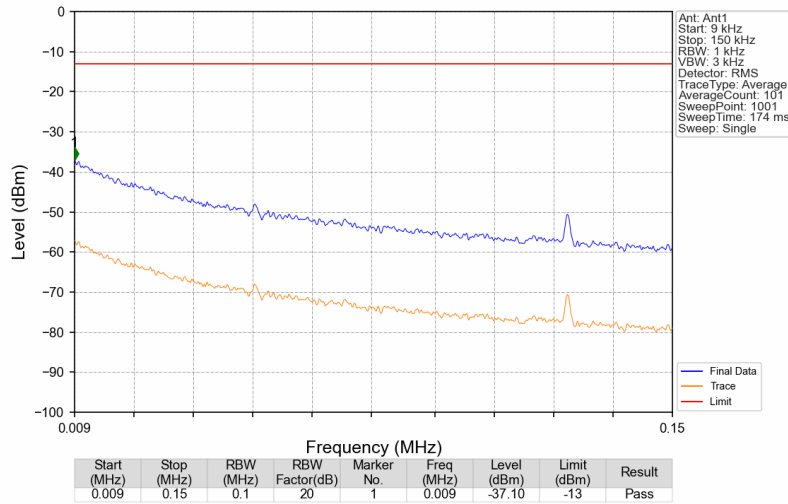
Band26a_859.1MHz_GMSK_SISO_Ant1_NTNV
