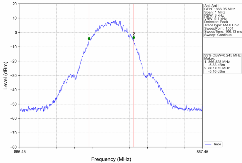
Band26a_866.95MHz_GMSK_SISO_Ant1_NTNV_AGC
