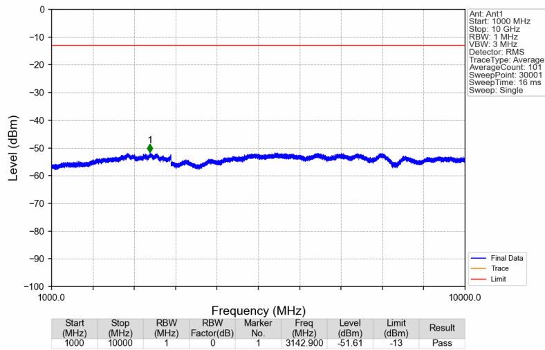
Band26a_859.1MHz_GMSK_SISO_Ant1_NTNV
