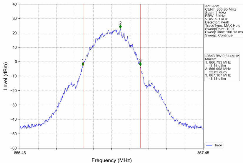
Band26a_866.95MHz_GMSK_SISO_Ant1_NTNV_AGC+3
