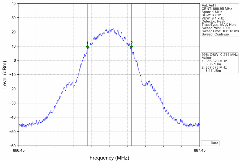
Band26a_866.95MHz_GMSK_SISO_Ant1_NTNV_AGC+3
