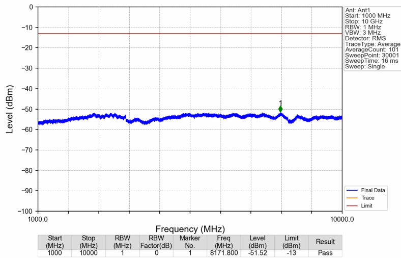
Band26a_866.5MHz_AWGN_SISO_Ant1_NTNV
