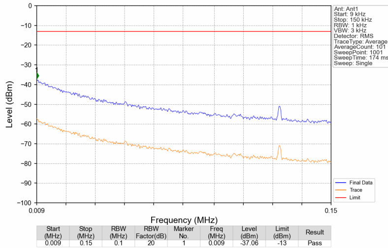
Band26a_866.5MHz_AWGN_SISO_Ant1_NTNV
