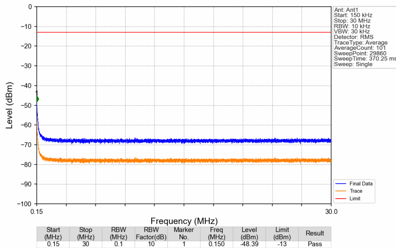
Band26a_868.9MHz_GMSK_SISO_Ant1_NTNV
