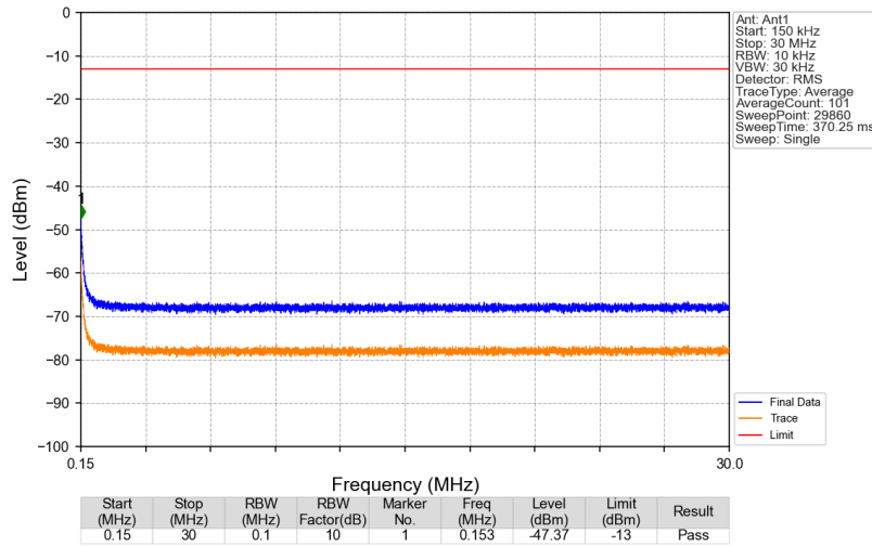
Band26a_859.1MHz_GMSK_SISO_Ant1_NTNV
