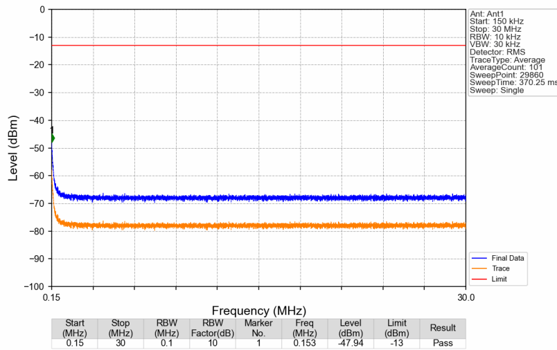
Band26a_866.5MHz_AWGN_SISO_Ant1_NTNV
