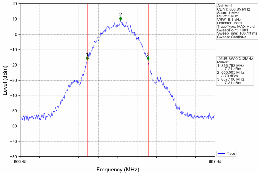
Band26a_866.95MHz_GMSK_SISO_Ant1_NTNV_AGC
