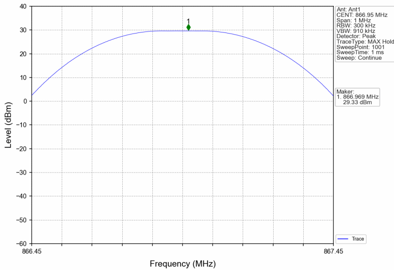
Band26a_866.95MHz_GMSK_SISO_Ant1_NTNV_AGC+3
