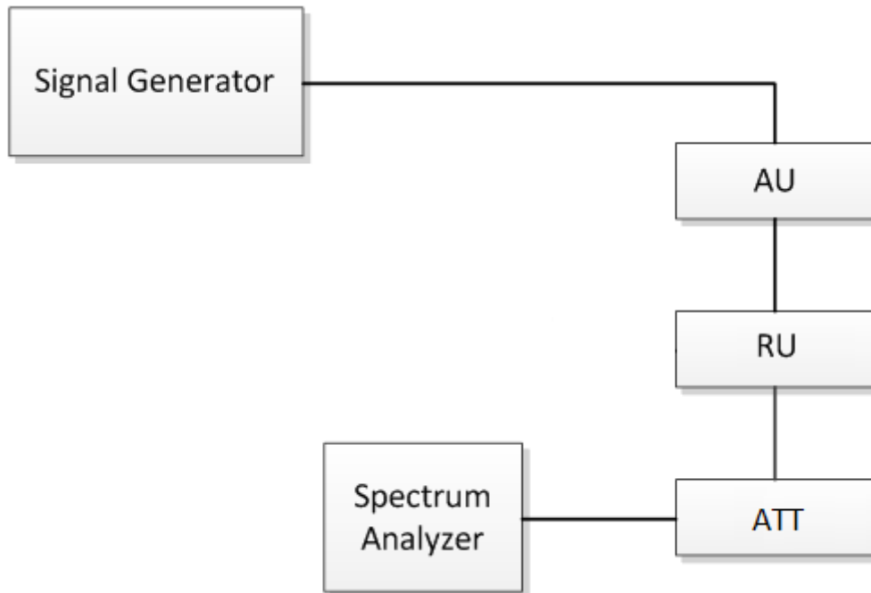
Fig.3. Band edge test configuration
