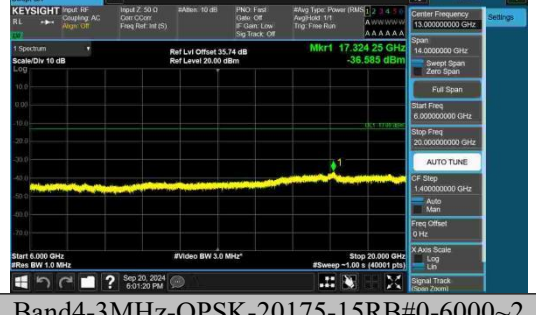
Band4-3MHz-QPSK-20175-15RB#0-6000~2 0000-PASS
