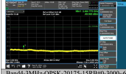
Band4-3MHz-QPSK-20175-15RB#0-3000~6 000-PASS
