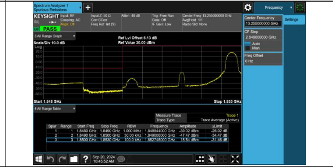
Band2-3MHz-QPSK-18615-1RB#14-PASS
