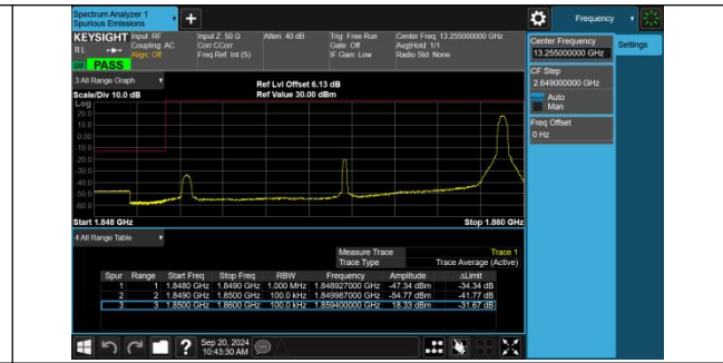
Band2-10MHz-QPSK-18650-1RB#49-PASS
