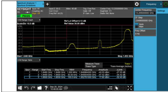
Band2-3MHz-16QAM-18615-1RB#14-PASS
