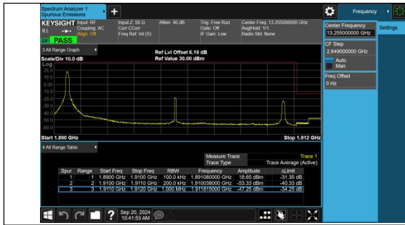
Band2-20MHz-QPSK-19100-1RB#0-PASS
