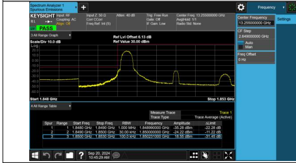
Band2-3MHz-QPSK-18615-1RB#0-PASS
