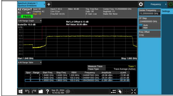
Band2-10MHz-QPSK-18650-50RB#0-PASS
