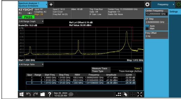
Band2-20MHz-16QAM-19100-1RB#99-PASS
