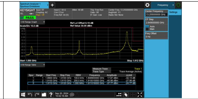
Band2-20MHz-QPSK-19100-1RB#99-PASS
