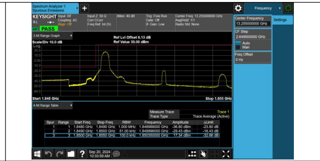
Band2-5MHz-16QAM-18625-1RB#0-PASS
