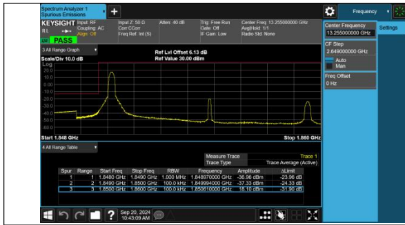
Band2-10MHz-QPSK-18650-1RB#0-PASS
