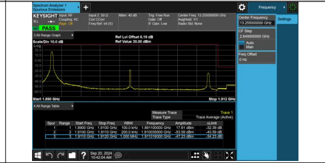
Band2-20MHz-16QAM-19100-1RB#0-PASS
