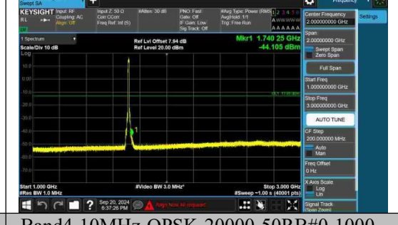
Band4-10MHz-QPSK-20000-50RB#0-1000~3000-PASS
