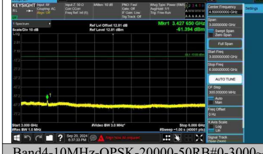
Band4-10MHz-QPSK-20000-50RB#0-3000~6000-PASS
