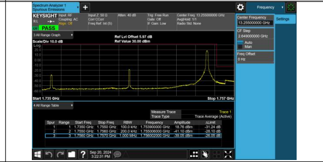
Band4-20MHz-QPSK-20300-1RB#99-PASS
