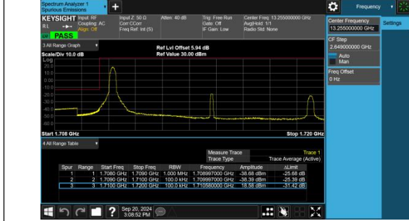
Band4-10MHz-QPSK-20000-1RB#0-PASS
