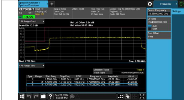
Band4-10MHz-QPSK-20000-50RB#0-PASS
