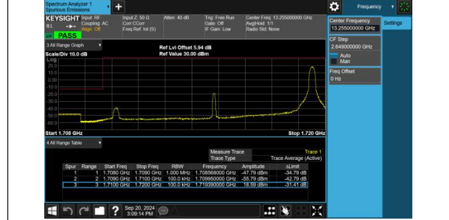
Band4-10MHz-QPSK-20000-1RB#49-PASS
