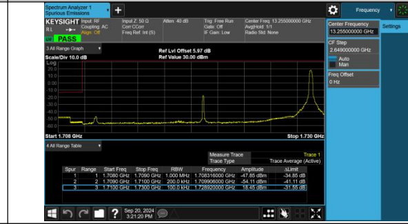
Band4-20MHz-QPSK-20050-1RB#99-PASS
