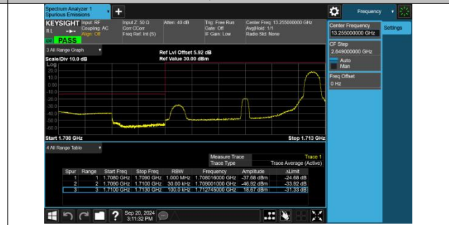
Band4-3MHz-QPSK-19965-1RB#14-PASS
