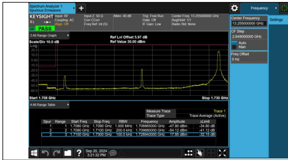
Band4-20MHz-16QAM-20050-1RB#99-PASS
