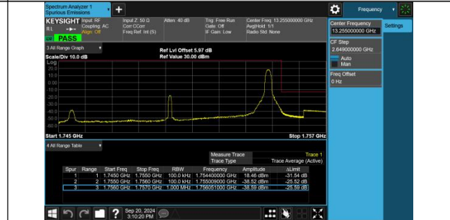
Band4-10MHz-QPSK-20350-1RB#49-PASS
