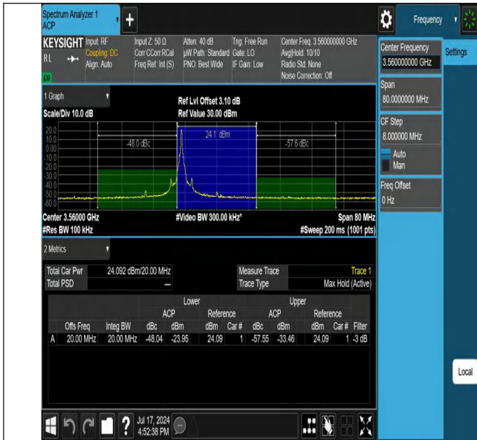
Band48-20MHz-QPSK-55340-1RB#0-PASS
