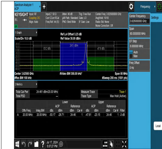
Band48-20MHz-QPSK-55990-1RB#99-PASS
