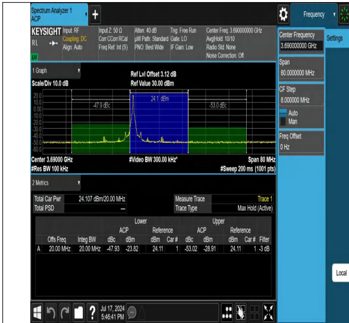
Band48-20MHz-QPSK-56640-1RB#0-PASS
