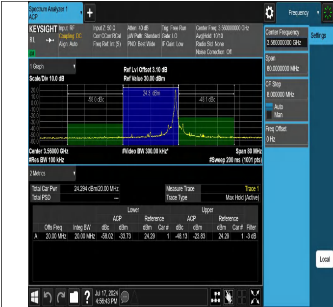
Band48-20MHz-QPSK-55340-1RB#99-PASS
