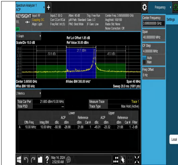
Band48-10MHz-QPSK-56690-1RB#49-PASS
