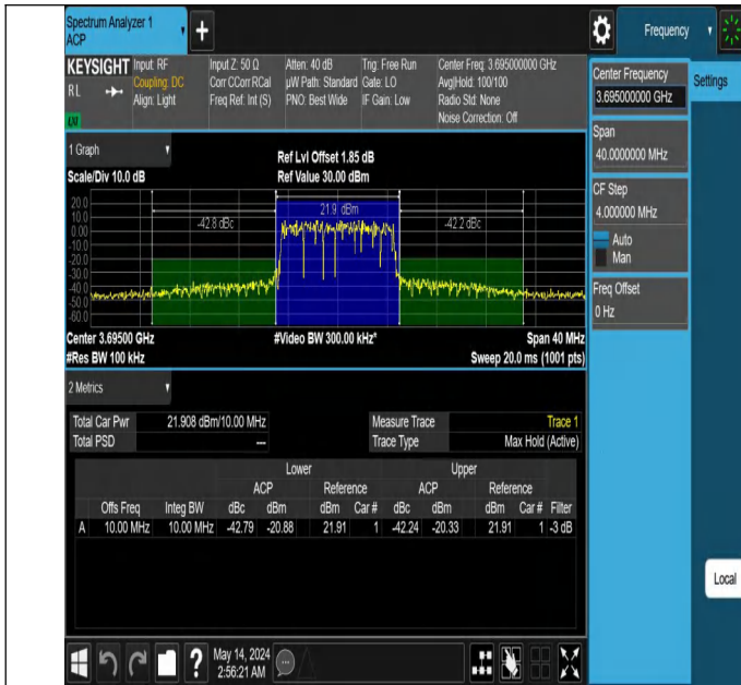
Band48-10MHz-QPSK-56690-50RB#0-PASS
