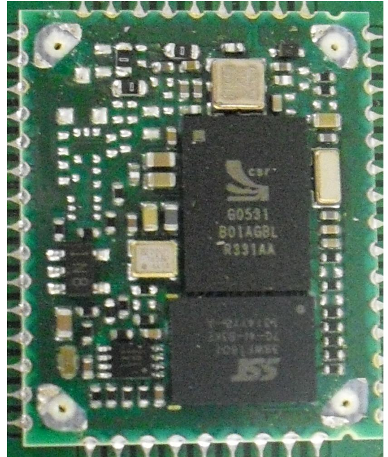
Module2 GNSS Module
