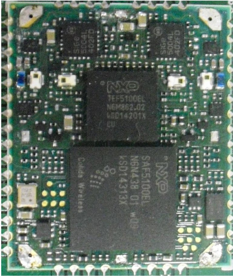
Module1 V2X Module
