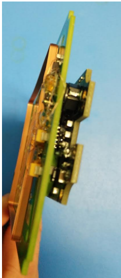
Bottom PCB
