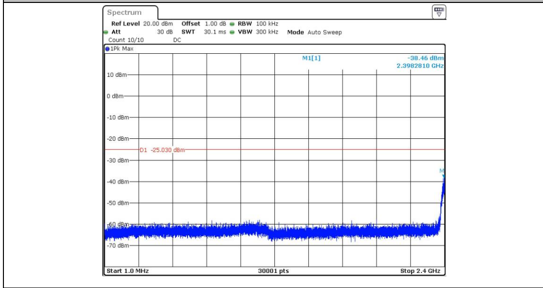
11N40_Ant1_2422_1~2400
