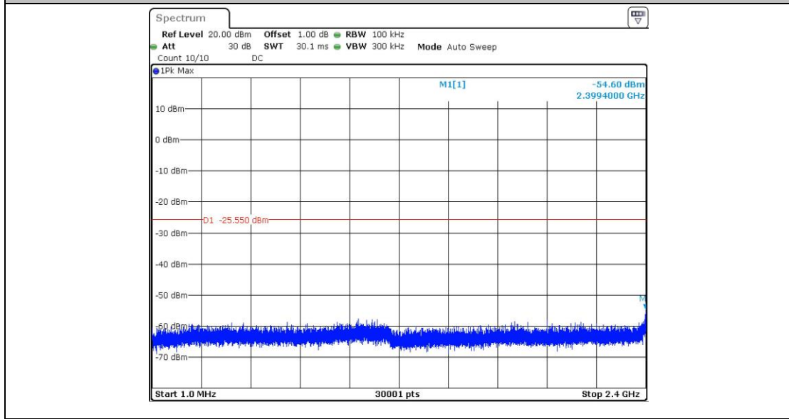
11N40_Ant1_2452_1~2400
