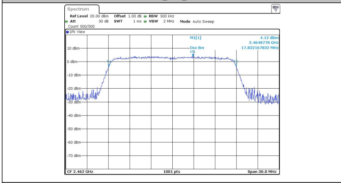
11N20_Ant1_2462
