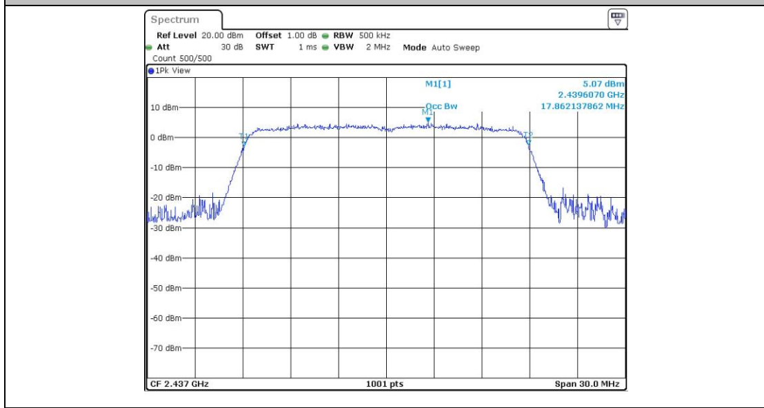
11N20_Ant1_2437
