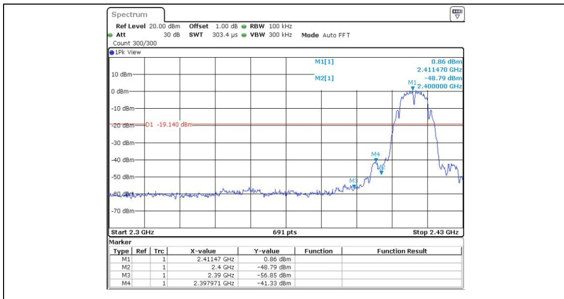
11B_Ant1_Low_2412
