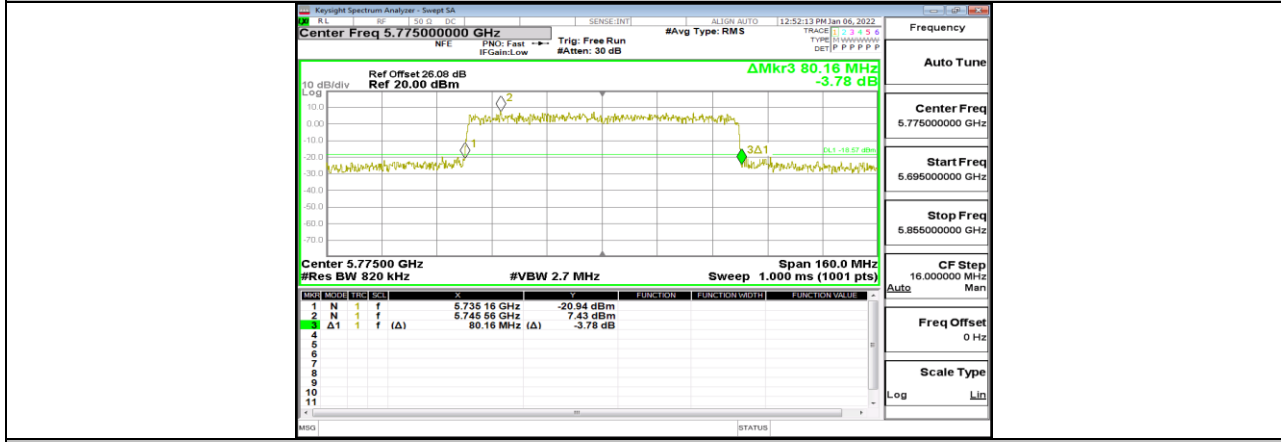
11AX80MIMO_Ant2_5775
