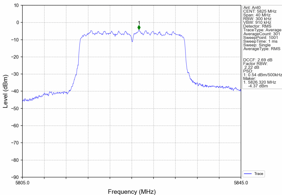
802.11ax(HEW20)_HCH_5825MHz_RU242_Left_Ant0_NTNV
