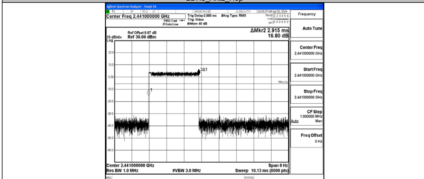
2DH5_Ant1_Hop
