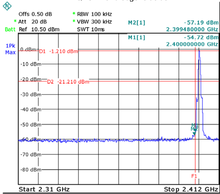
Pi/4 DQPSK Band edge-left side
