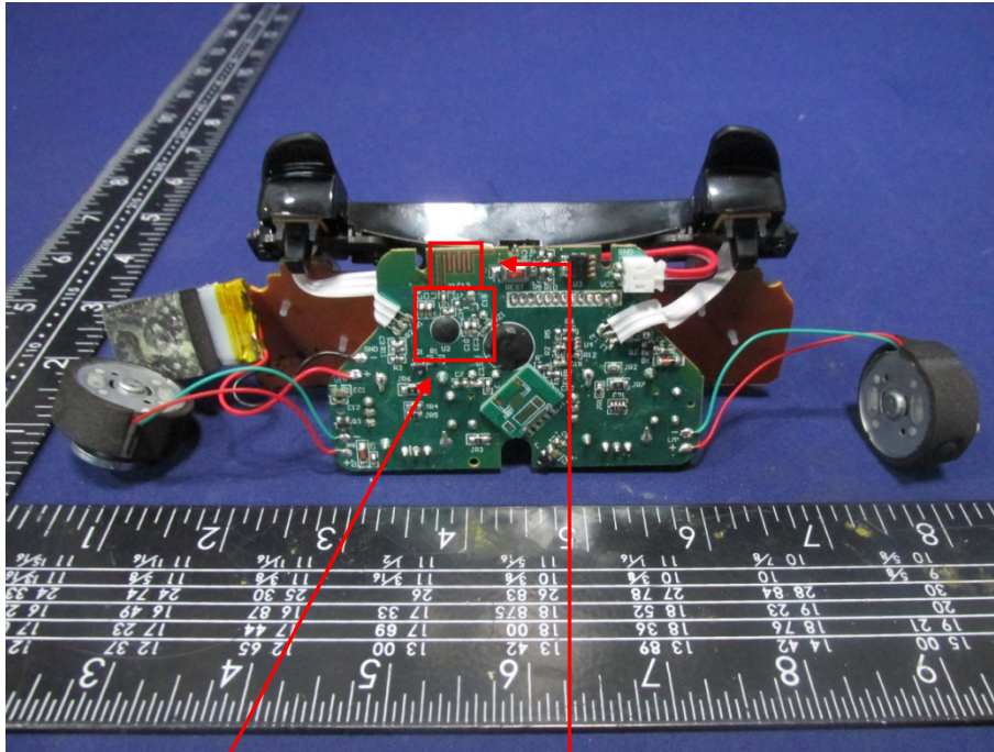
2.4G module
