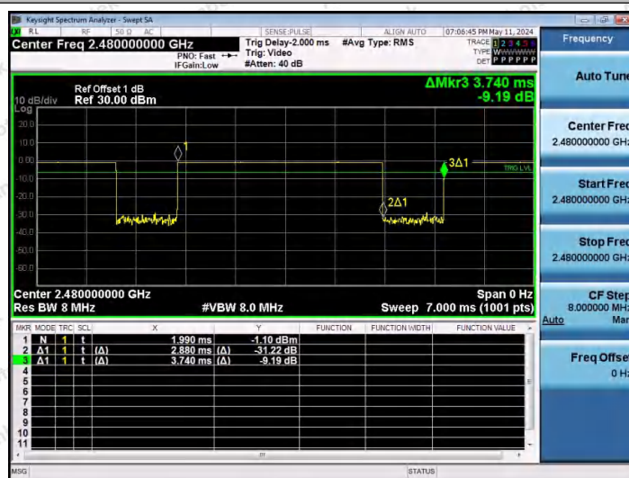
NTNV-DH5-Ant1-2480
