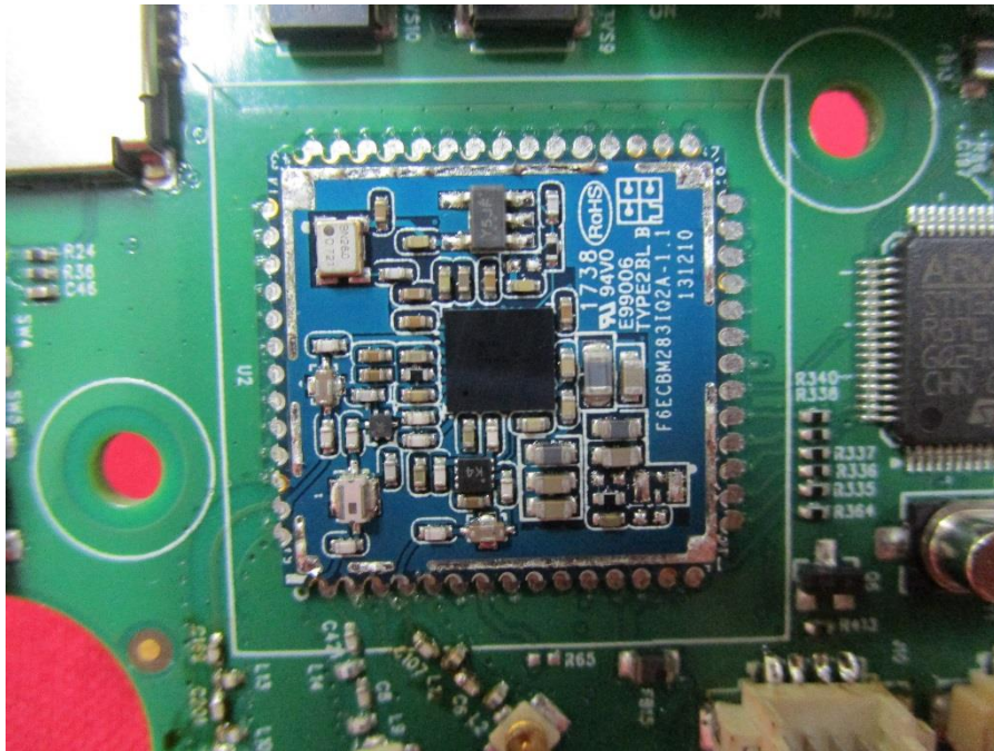
WIFI module
