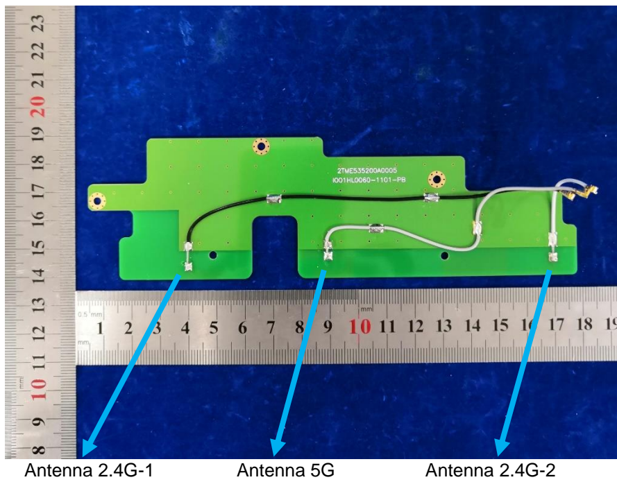
ANTENNA
