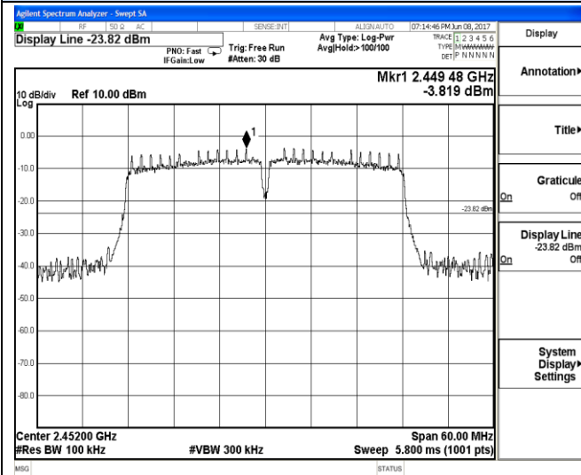
2422 MHz – 2482 MHz
