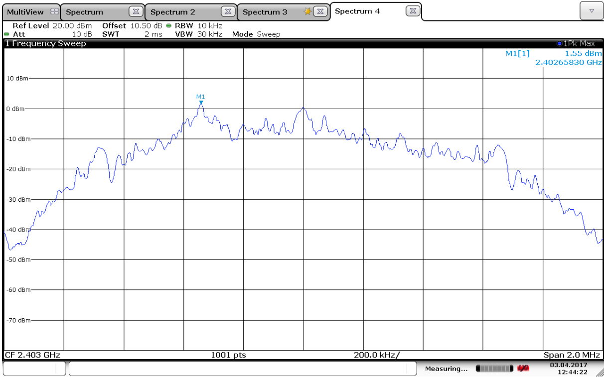
PSD, 2403MHz
