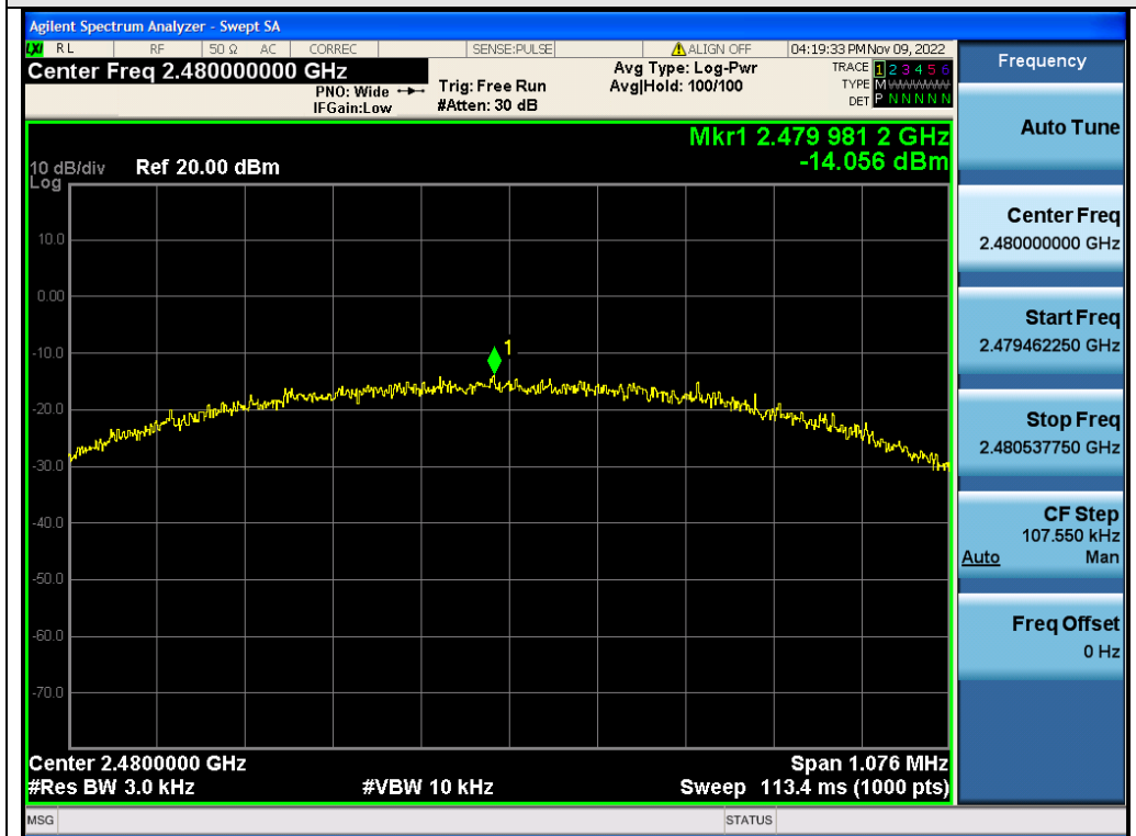
Test_Graph_2.4G_ANT2_2480_1Mbps_PSD
