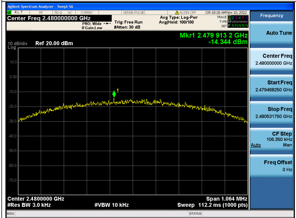
Test_Graph_GFSK_ANT2_2480_PSD
