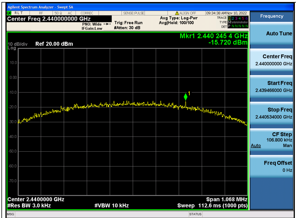
Test_Graph_GFSK_ANT2_2440_PSD
