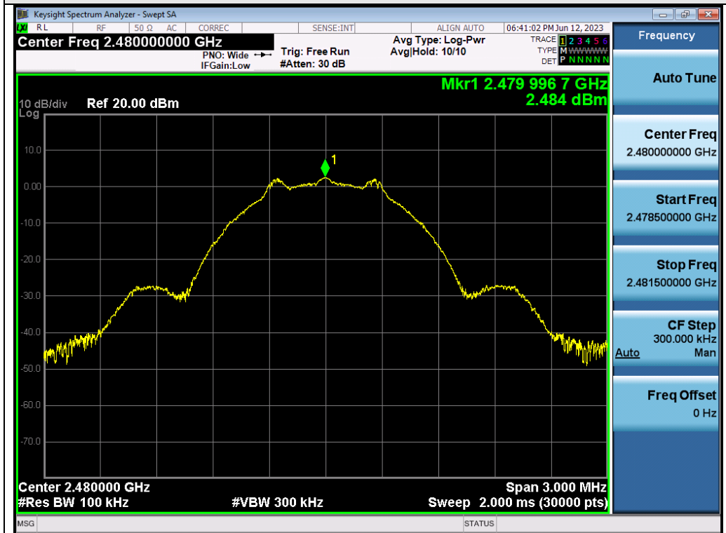
Test_Graph_ANT2_2480_Reference Level
