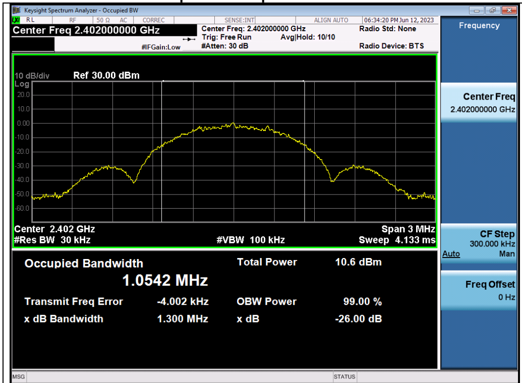
Test_Graph_ANT2_2402_OBW
