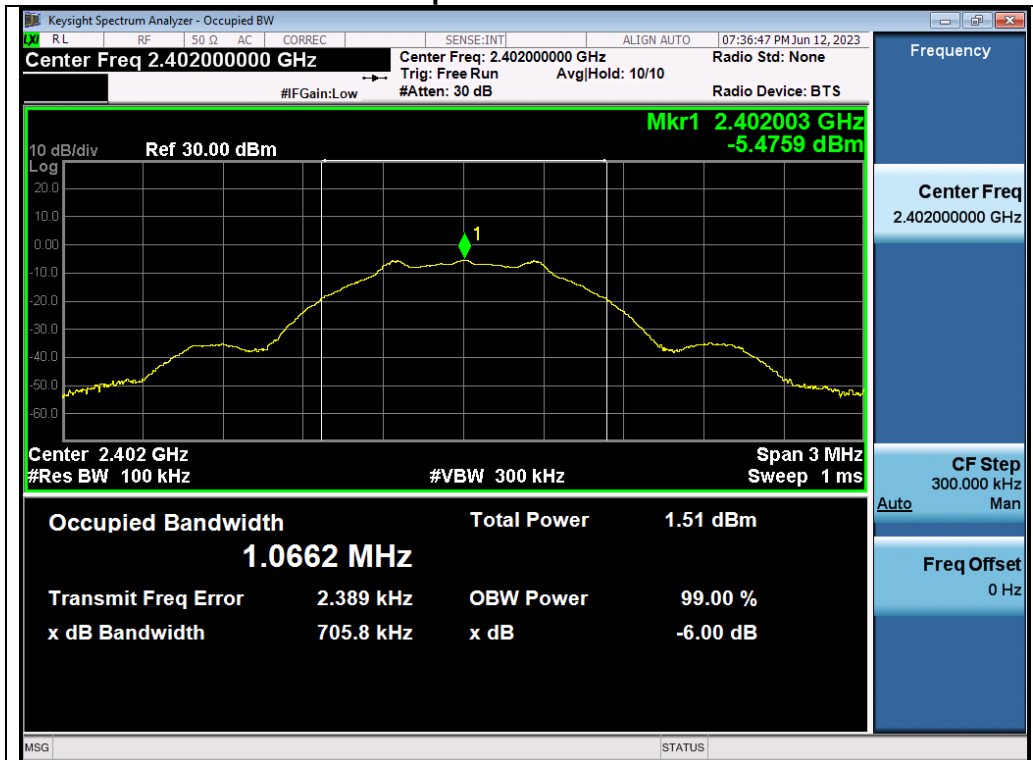
Test_Graph_ANT1_2402_DTSBW
