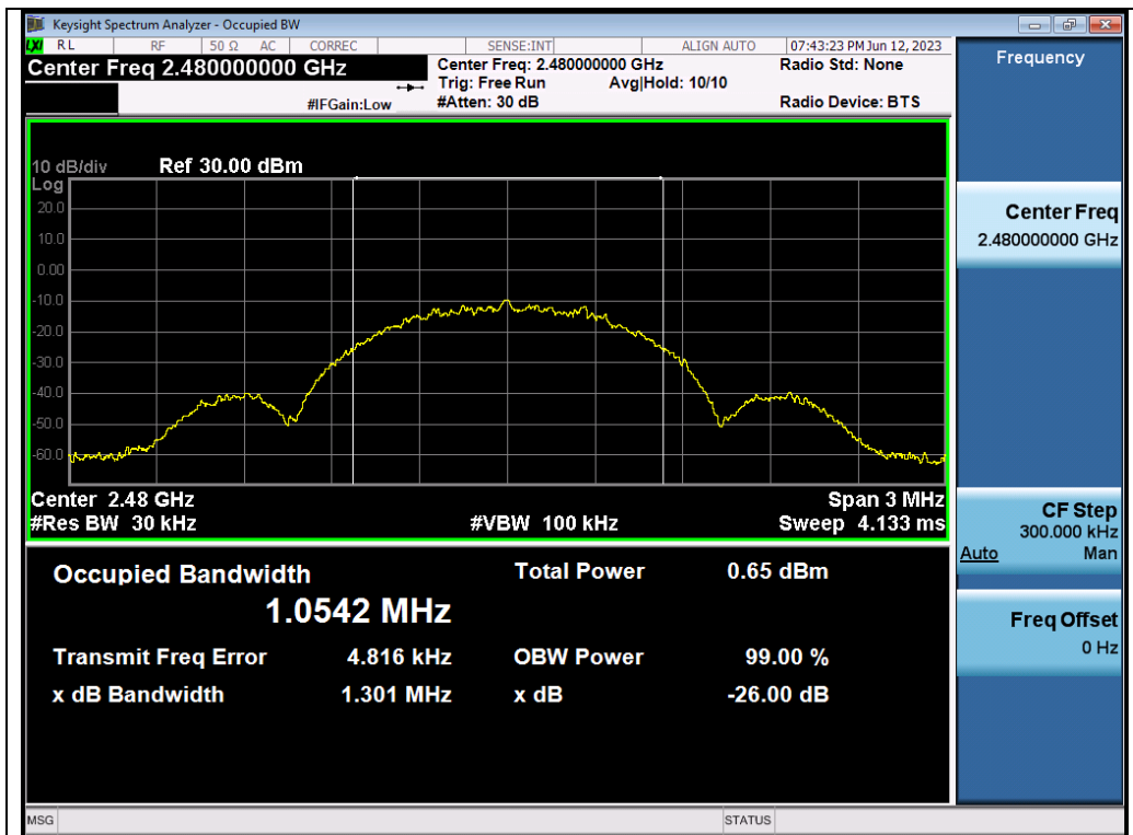
Test_Graph_ANT1_2480_OBW
