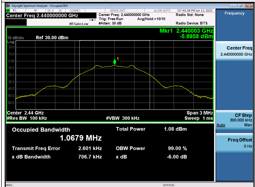
Test_Graph_ANT1_2440_DTSBW
