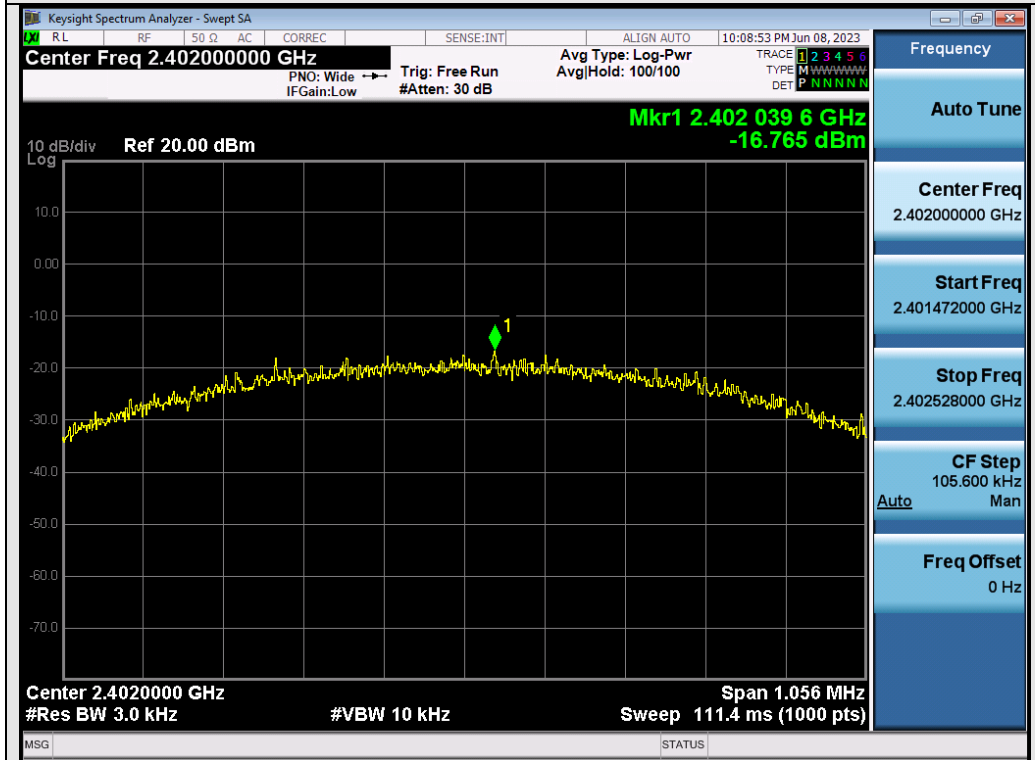
Test_Graph_ANT2_2402_PSD
