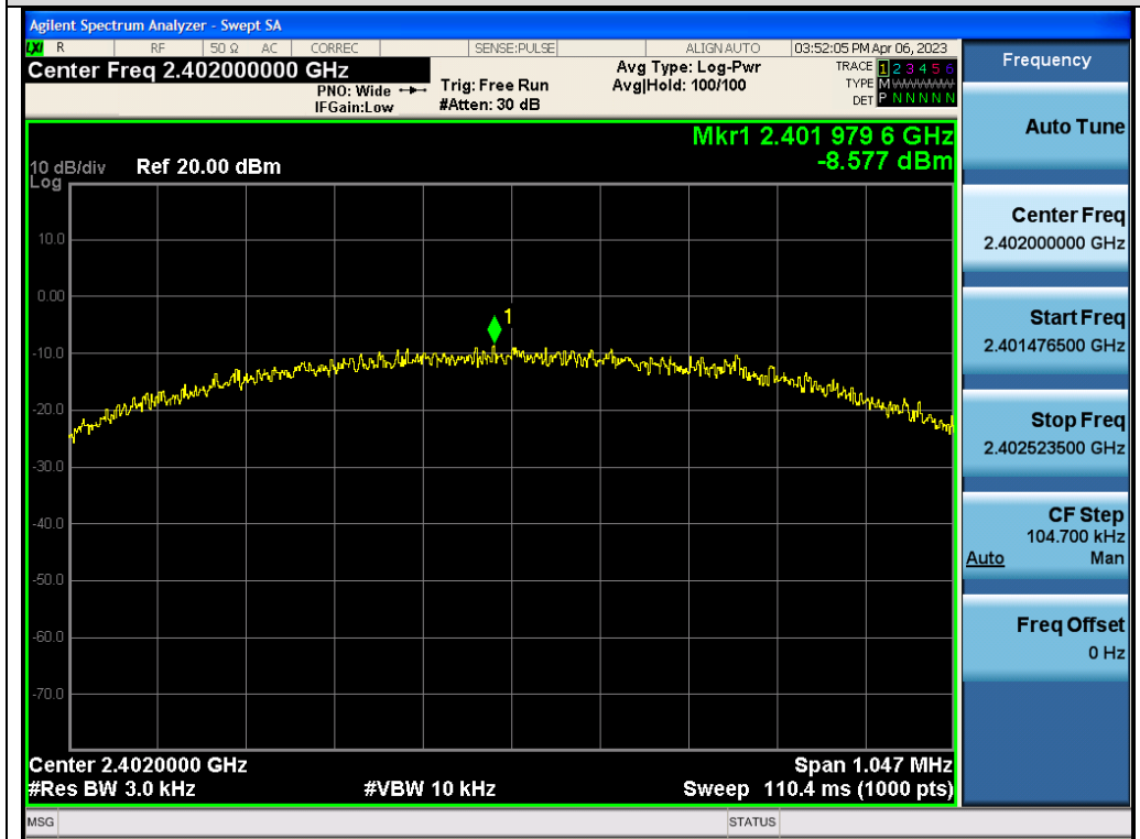
Test_Graph_LE1M_ANT2_2402_1Mbps_PSD
