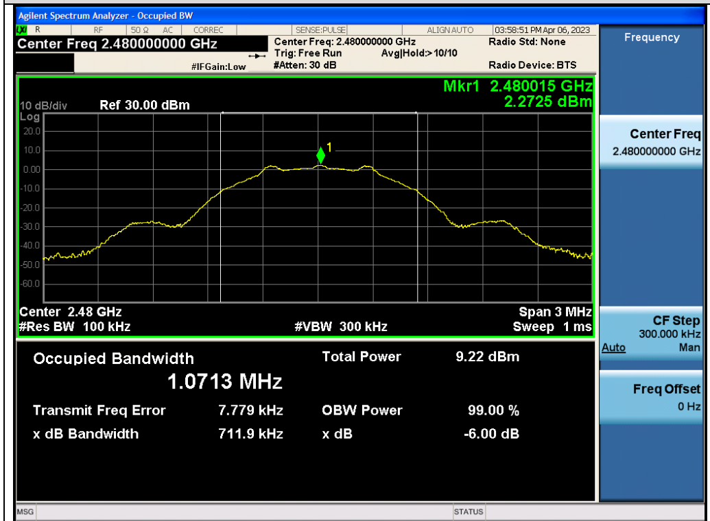
Test_Graph_LE1M_ANT2_2480_1Mbps_DTSBW
