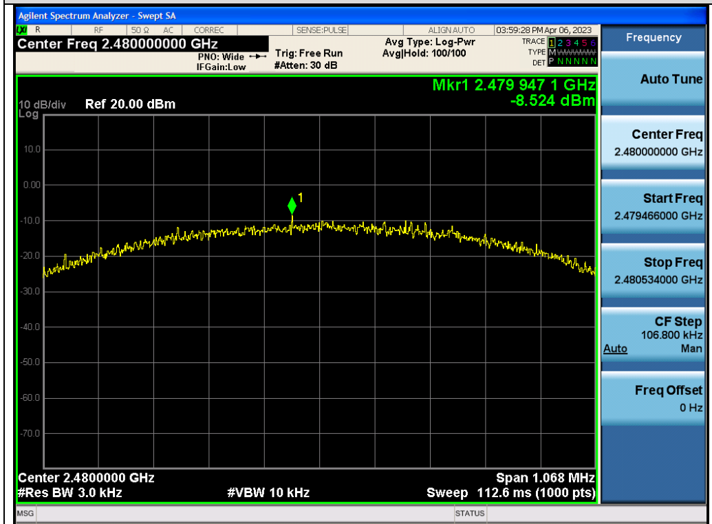
Test_Graph_LE1M_ANT2_2480_1Mbps_PSD
