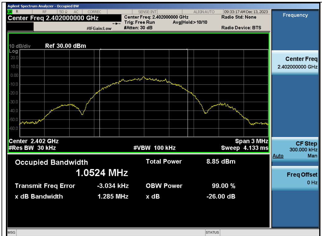
Test_Graph_GFSK_ANT2_2402_OBW
