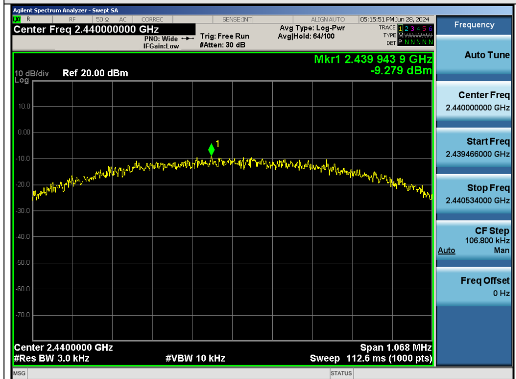
Test_Graph_GFSK_ANT2_2440_PSD
