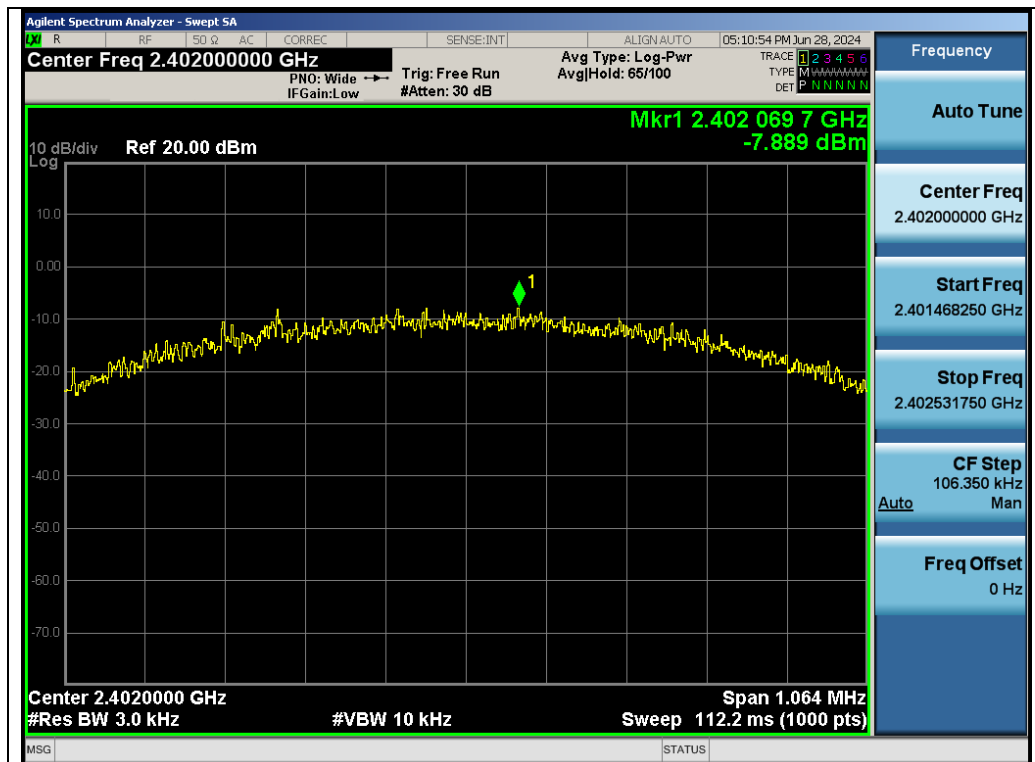
Test_Graph_GFSK_ANT2_2402_PSD
