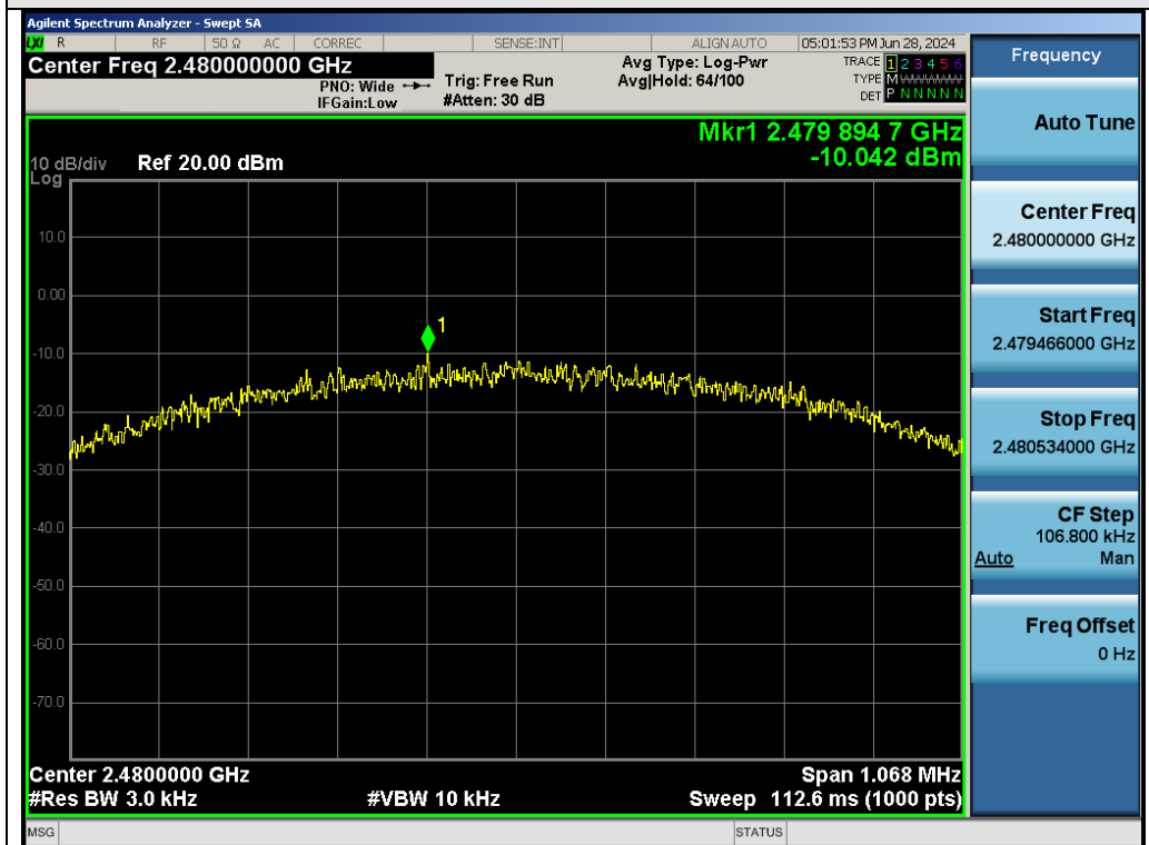
Test_Graph_GFSK_ANT1_2480_PSD
