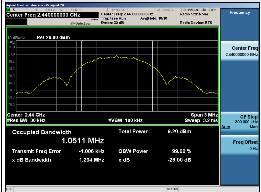
Test_Graph_GFSK_ANT2_2440_OBW
