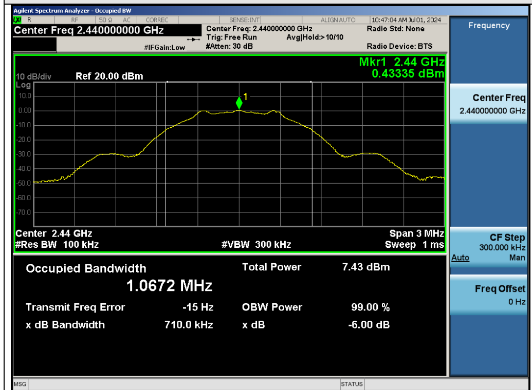
Test_Graph_GFSK_ANT2_2440_DTSBW
