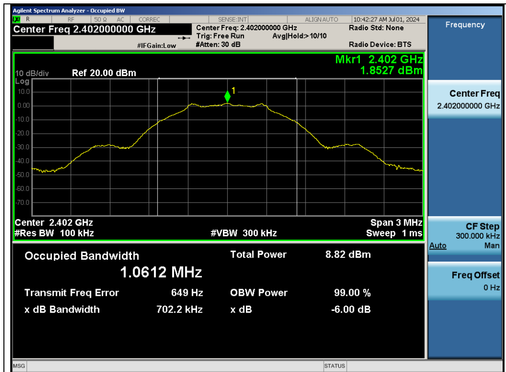
Test_Graph_GFSK_ANT2_2402_DTSBW
