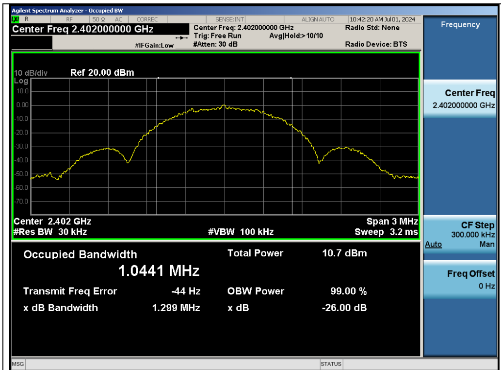
Test_Graph_GFSK_ANT2_2402_OBW
