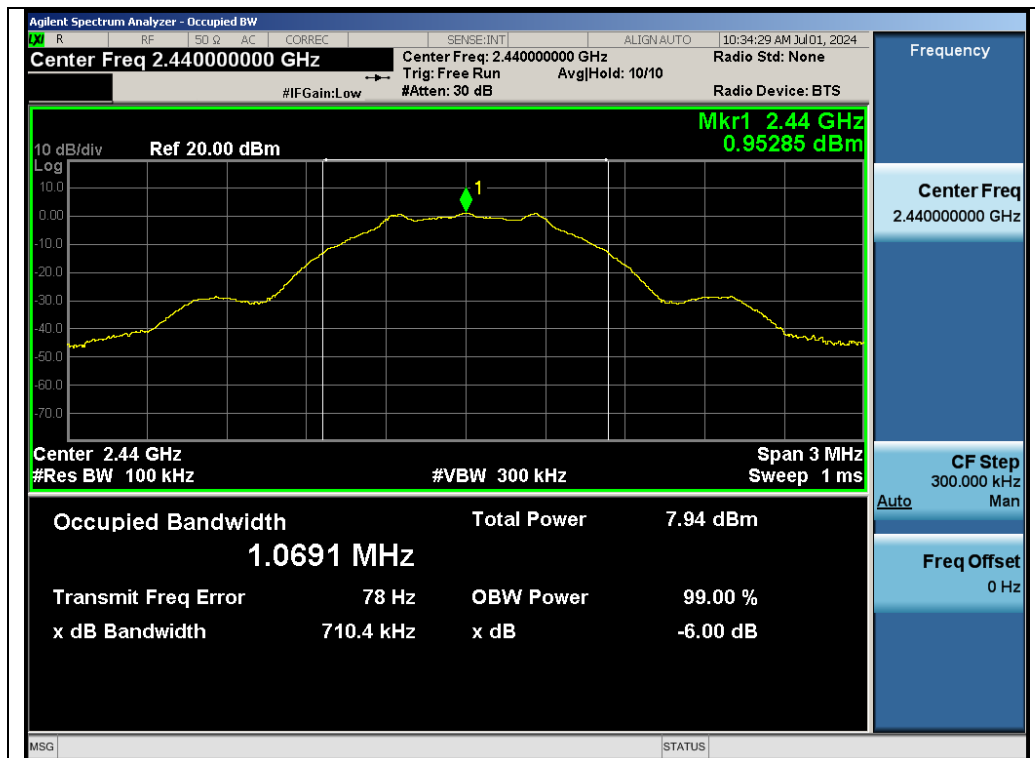
Test_Graph_GFSK_ANT1_2440_DTSBW
