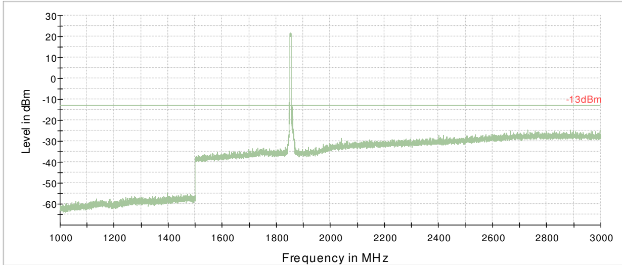
PK+_CLRWR@1GHz-3GHz B2 LOW CH -13dBm
